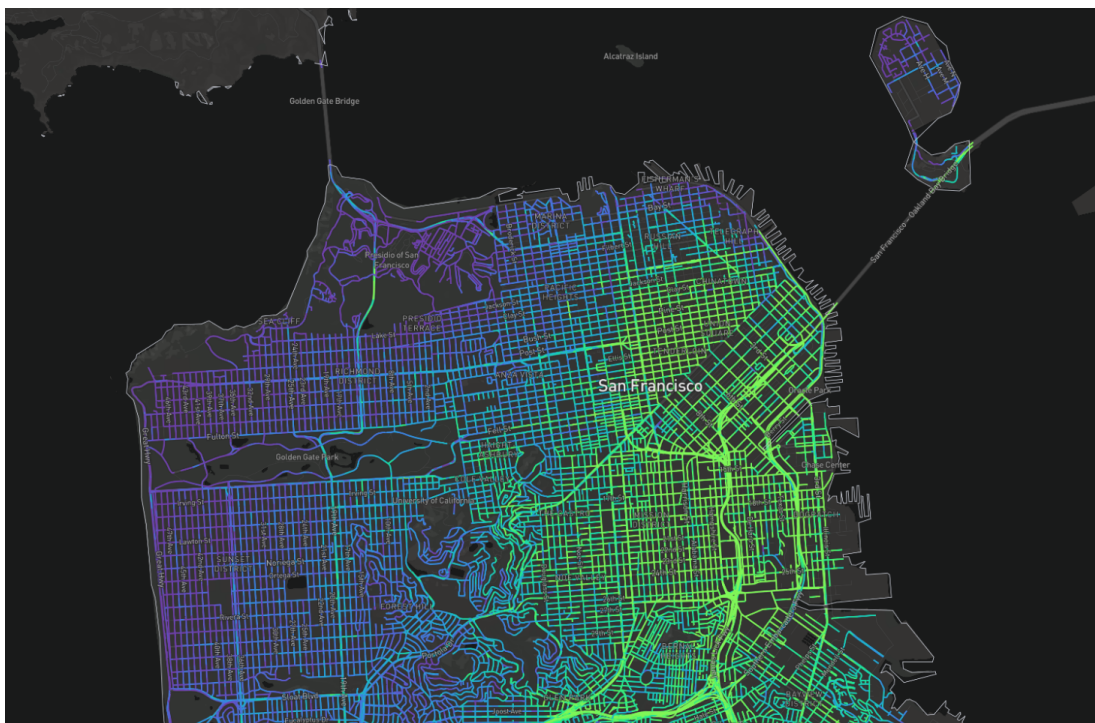
Figura 2: Ejemplo de estimaciones de concentración ambiental graficadas para el NO2 (dióxido de nitrógeno) en el Área de la Bahía de San Francisco, CA. Este gráfico utiliza datos generados por el método de monitoreo de área amplia.
