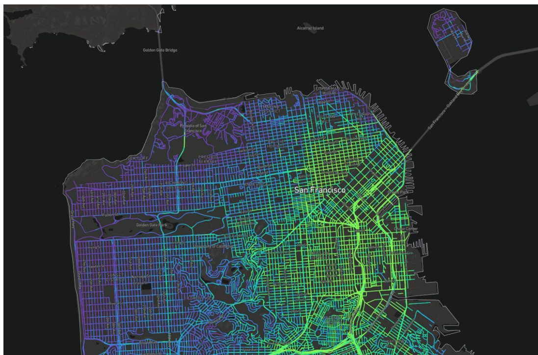
Figura 3: Ejemplo de estimaciones de concentración ambiental graficadas para el NO2 (dióxido de nitrógeno) en el Área de la Bahía de San Francisco, CA. Este gráfico utiliza datos generados por el método de monitoreo de área amplia.
